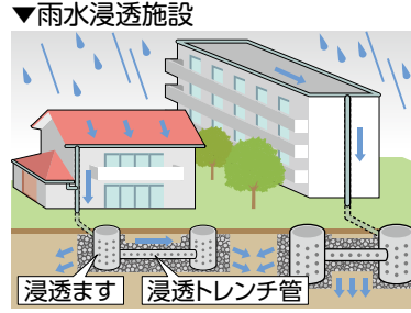
穴あきのます(浸透ます)と穴あきの排水管(浸透トレンチ管)を組み合わせで浸透させます。
